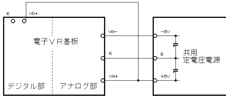
2電源 デジタル、アナログ共用電源の場合
